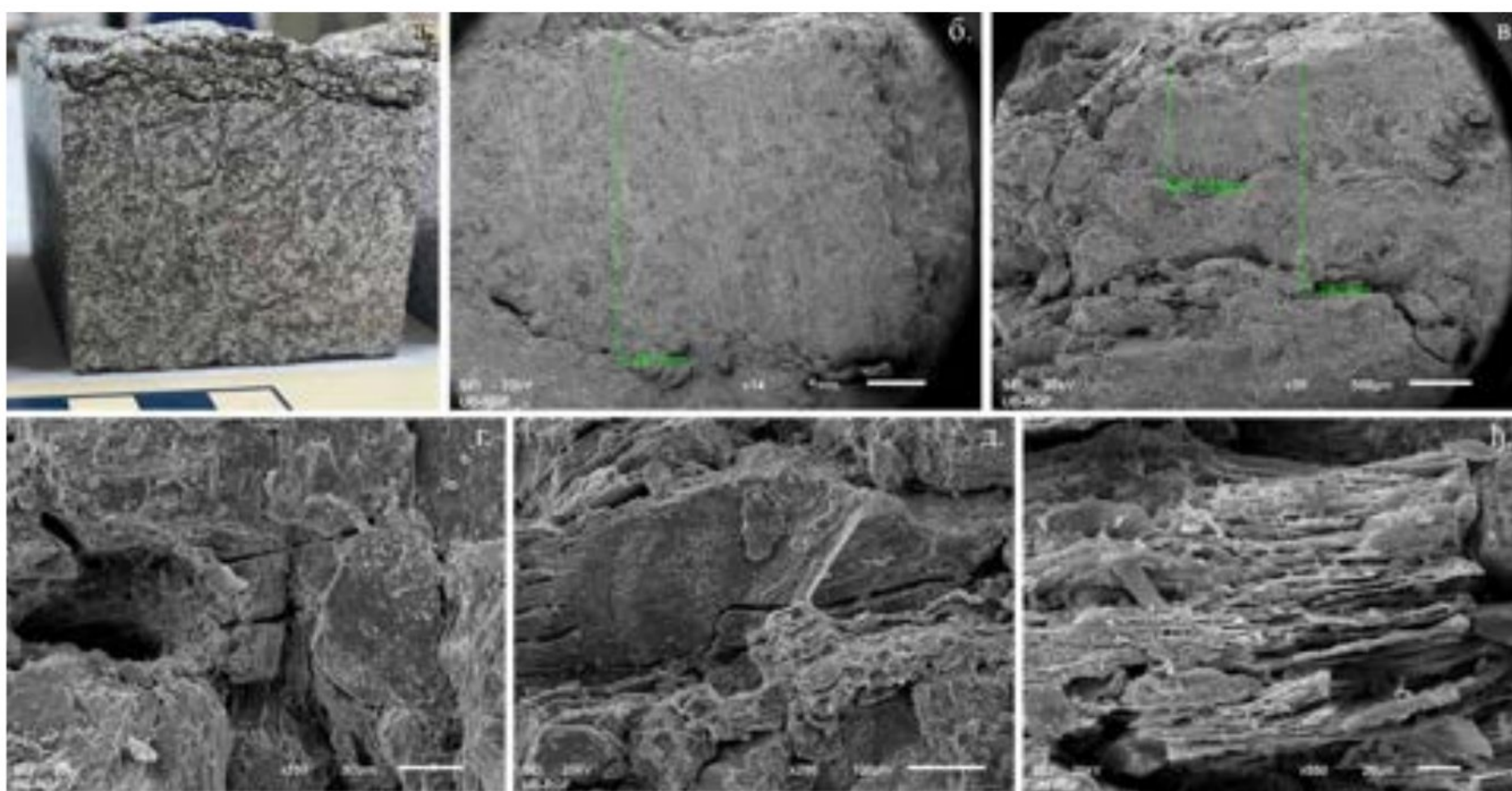
Слика 117. Приказ оштећења на узорку 25 MS а) макроскопски изглед узорка 25 MS; б-в) SEM снимци микропрелина површински ослабљене зоне камена; г) SEM снимак зоне са видљивим капиларним порема створеним штоковањем; д-ђ) SEM снимак микро фрактурисаних минерала керсантита.
