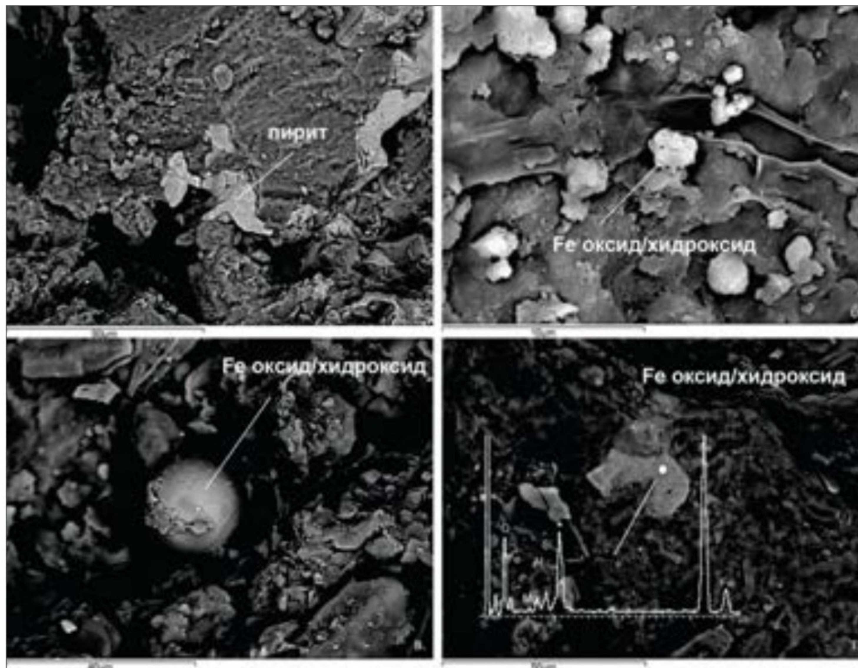
Слика 105. SEM снимци морфологије гвожђевитих минерала у површинским корима уграђеног керсантита; а) пирит у узорку 8MS; б) неправилни зрнасти агрегати Fe оксида/хидроксида у узорку 4MS; в) сферична честица Fe оксида/хидроксида у узорку 4MS; г) неправилни агрегати Fe оксида/хидроксида у узорку 5MS
