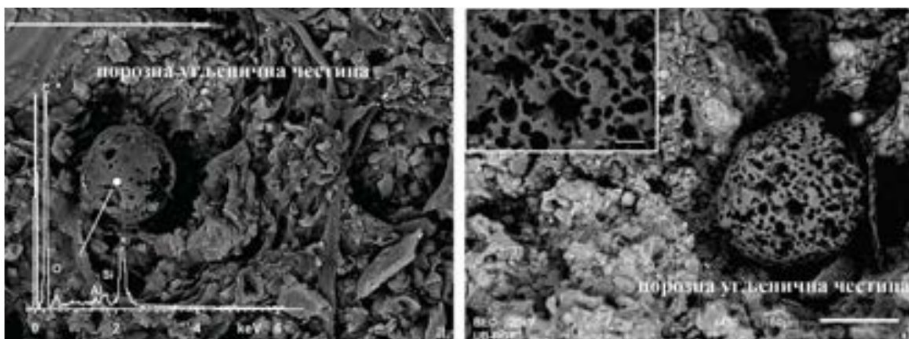
Слика 106. SEM снимци сфероидних честица а) порозна угљенична честица из узорка 13MS; в) порозна угљенична честица из узорка 9MS пречника 60 \mu\text{m} са величином пора до 10 \mu\text{m} (увеличан детаљ у горњем левом углу)
