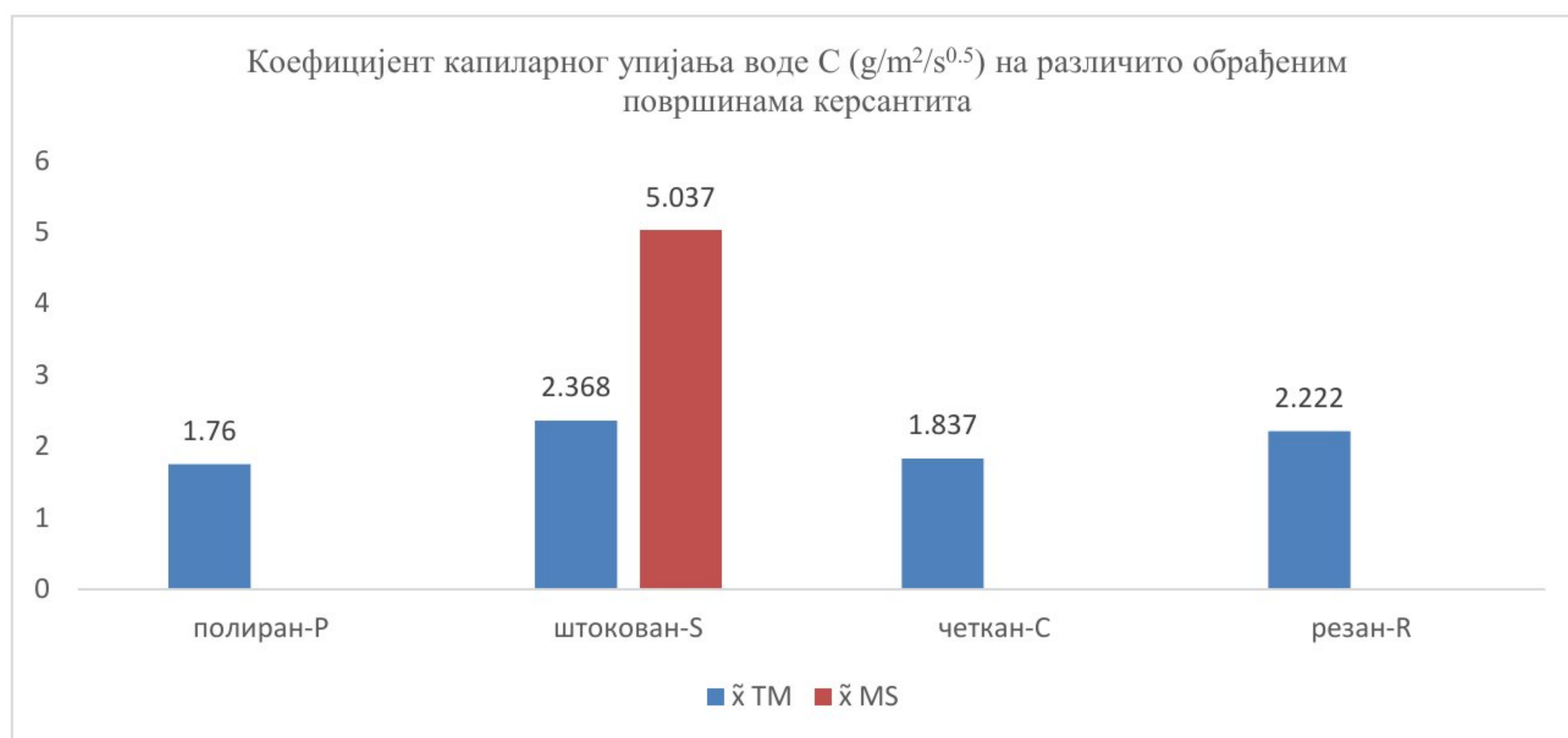
Слика 128. Хистограм средњих вредности коефицијента капиларног упијања воде различито површински обрађених површина и деградираних штокованих површина након стогодишње изложености атмосферијима
