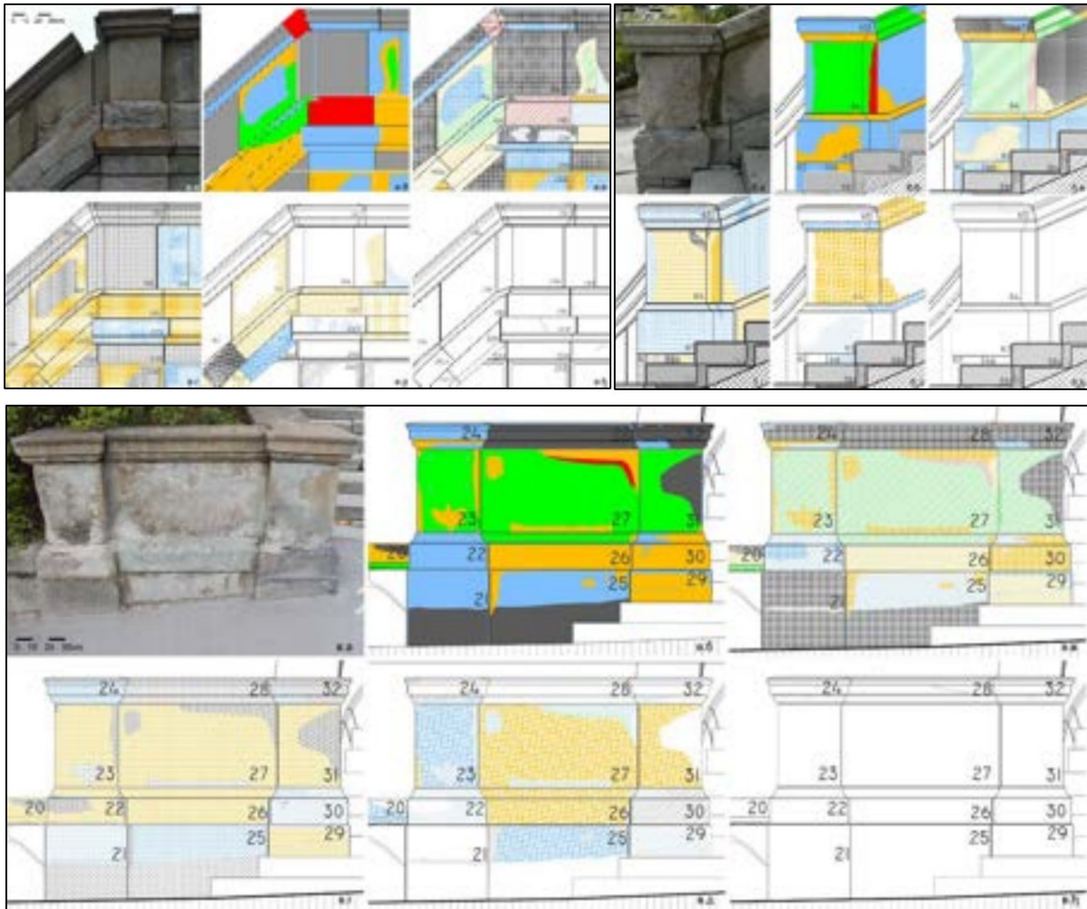
Слика 52. Приказ примера појединих делова објекта са графички приказаним обједињеним и појединачним групама оштећења: а) део централне лучне ограде а.а) фотографија стања а.б) приказ сумираних категорија оштећења а.в) мапа прве групе оштећења-губитак каменог материјала а.г) мапа друге групе оштећења-деколорација/наслаге а.д) мапа треће групе оштећења-одвајање а.е) мапа четврте групе оштећења-пукотине б) стуб ограде на подесту б.а) фотографија стања б.б) приказ сумираних категорија оштећења б.в) мапа прве групе оштећења-губитак каменог материјала б.г) мапа друге групе оштећења-деколорација/наслаге б.д) мапа треће групе оштећења-одвајање б.е) мапа четврте групе оштећења-пукотине в) леви доњи део ограде в.а) фотографија стања в.б) приказ сумираних категорија оштећења в.в) мапа прве групе оштећења-губитак каменог материјала в.г) мапа друге групе оштећења-деколорација/наслаге в.д) мапа треће групе оштећења-одвајање в.е) мапа четврте групе оштећења-пукотине
