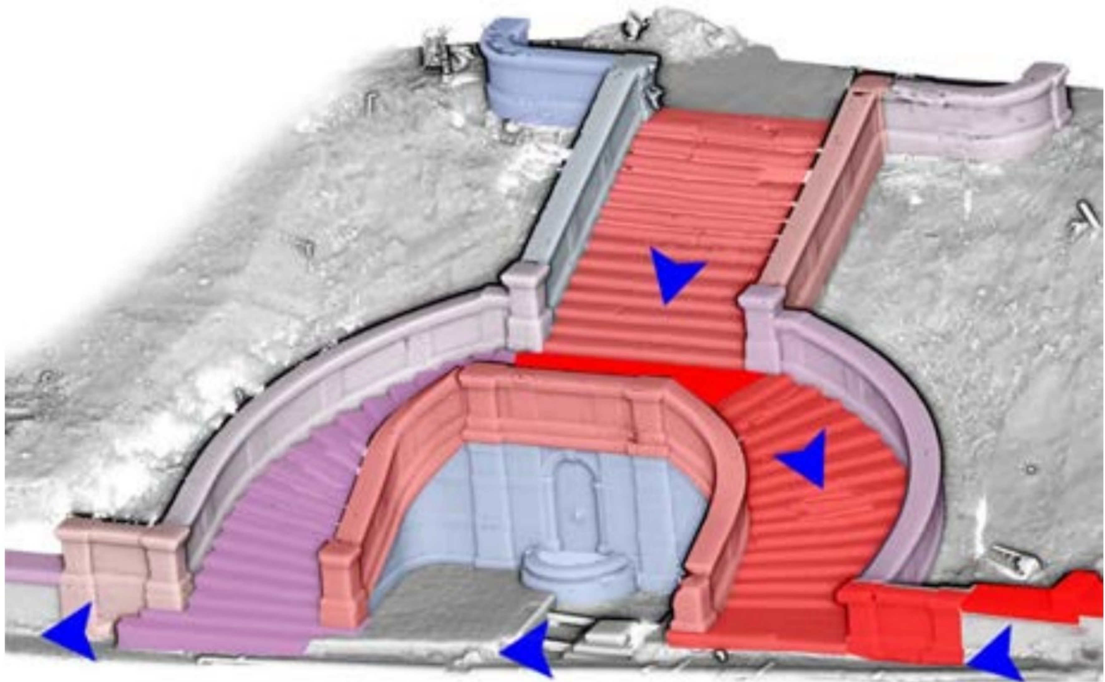
Слика 131.3Д Модел Малог степеништа са градираним бојама сегмента према интензитету вредности DI_{prog} (највећи интензитет – најјача црвена боја) и обележеним главним правцима кретања воде
