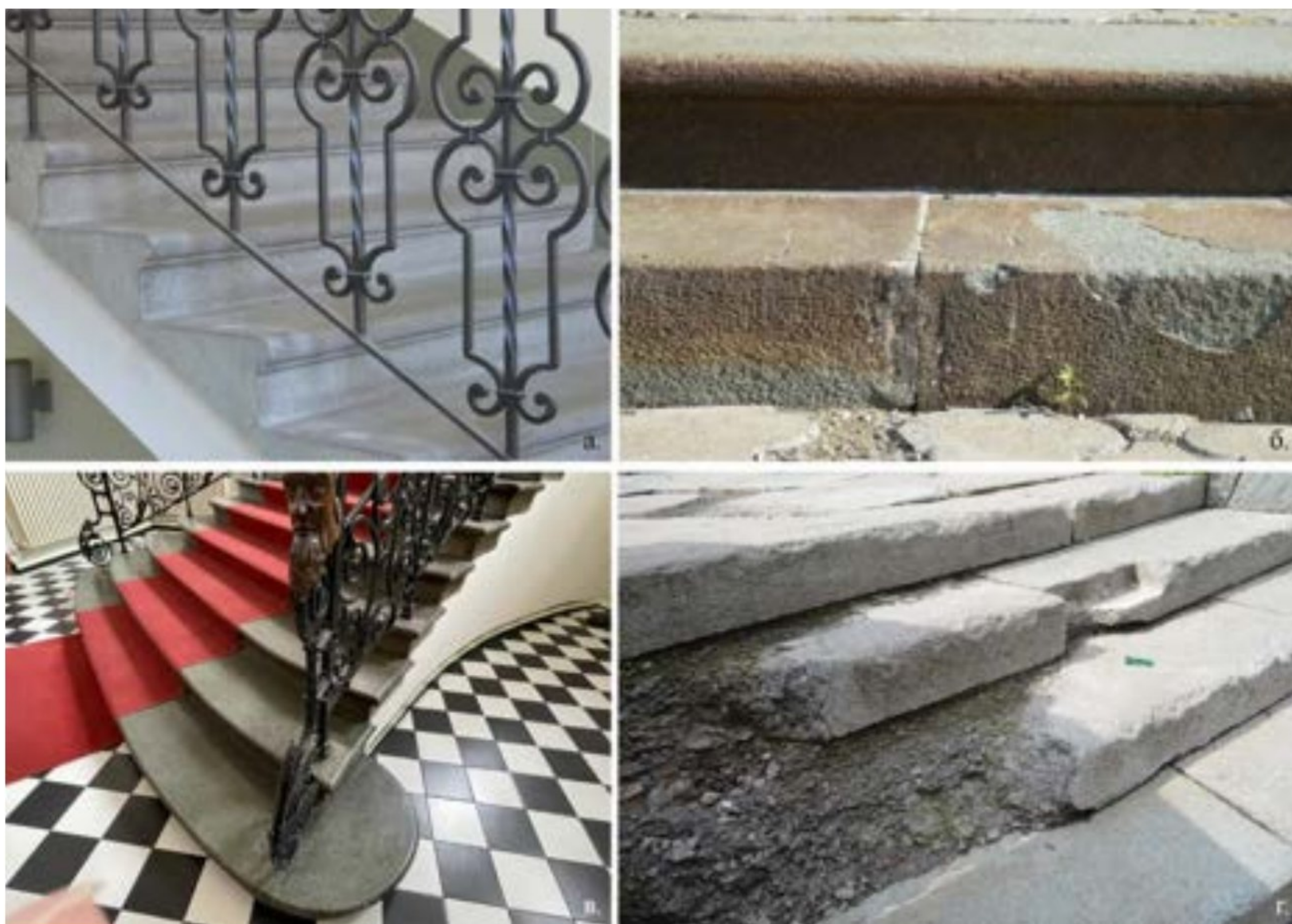
Слика 119. Степенице од керсантита: а) унутрашње степениште у Градском правобранилаштву; б) спољашње улазно степениште у Градском правобранилаштву; в) унутрашње степениште у згради Класне лутрије; г) део Малог степеништа
