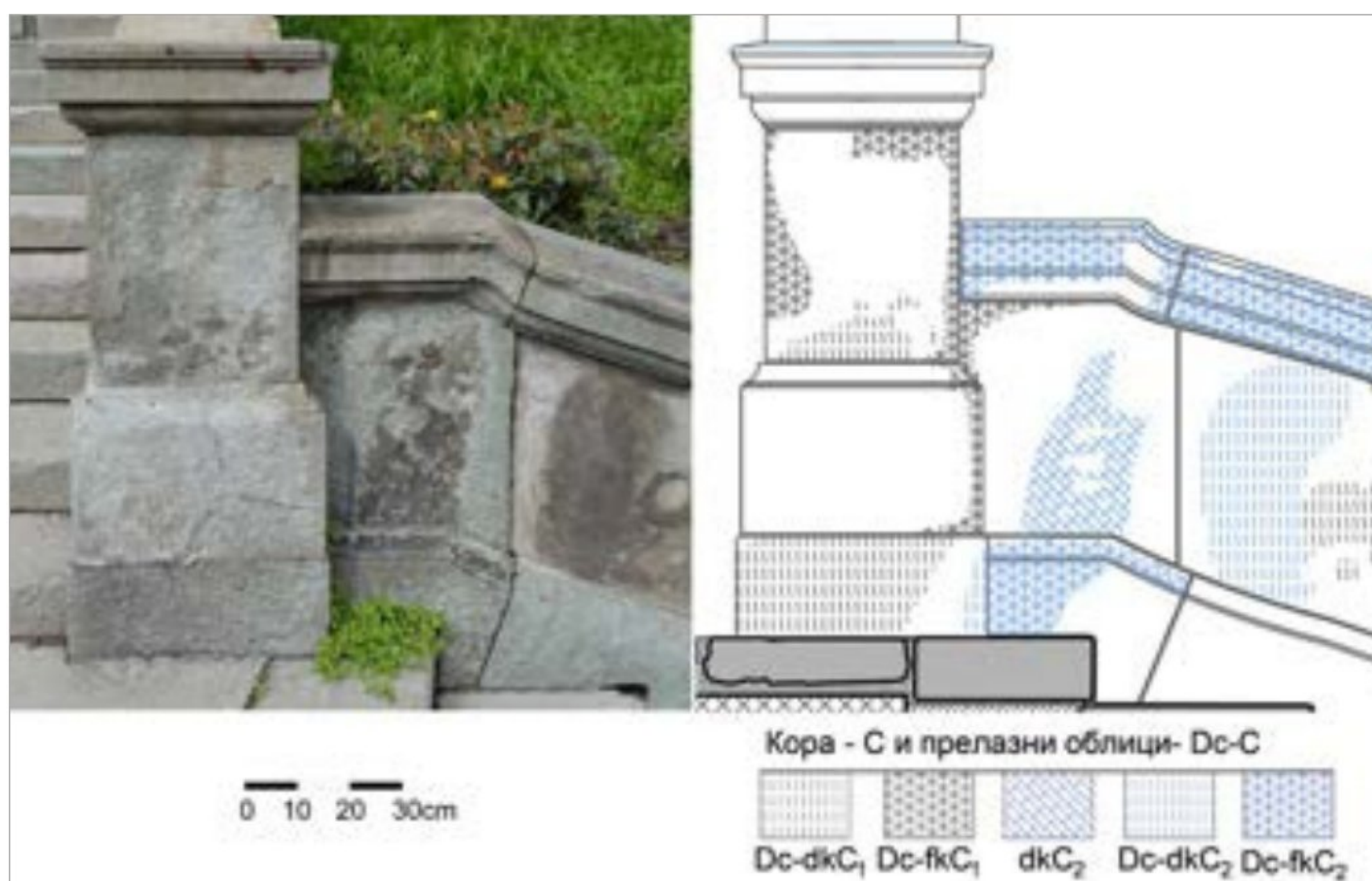
Слика 42. Коре: фотографија и графички приказ мапирања
