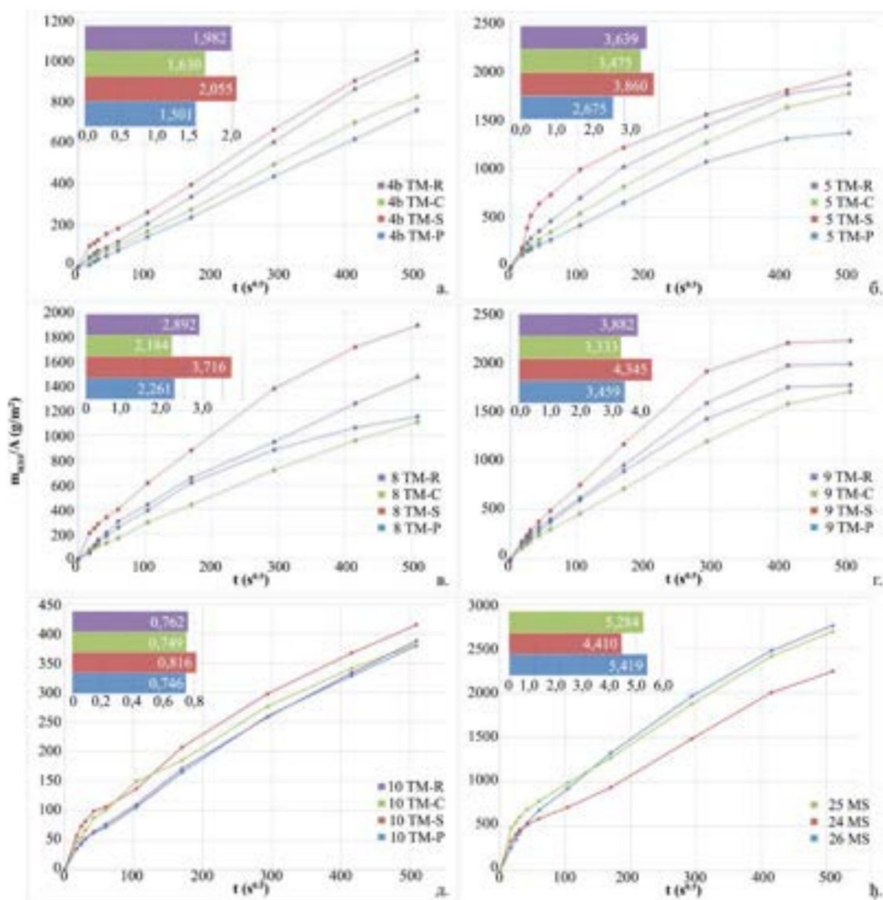
Слика 113. Графички приказ резултата капиларног упијања воде узорка керсантита из каменолома и узорка површински деградираниог керсантита са Малог степеништа; хистограм коефицијента капиларног упијања воде (C) (горњи леви угао дијаграма) и криве капиларног упијања керсантита узорка 4bTM (а) и узорка 5TM (б), узорка 8TM (в), узорка 9TM (г), узорка 10TM (д) и узорка са Малог степеништа 24MS, 25MS и 26MS (ж)
