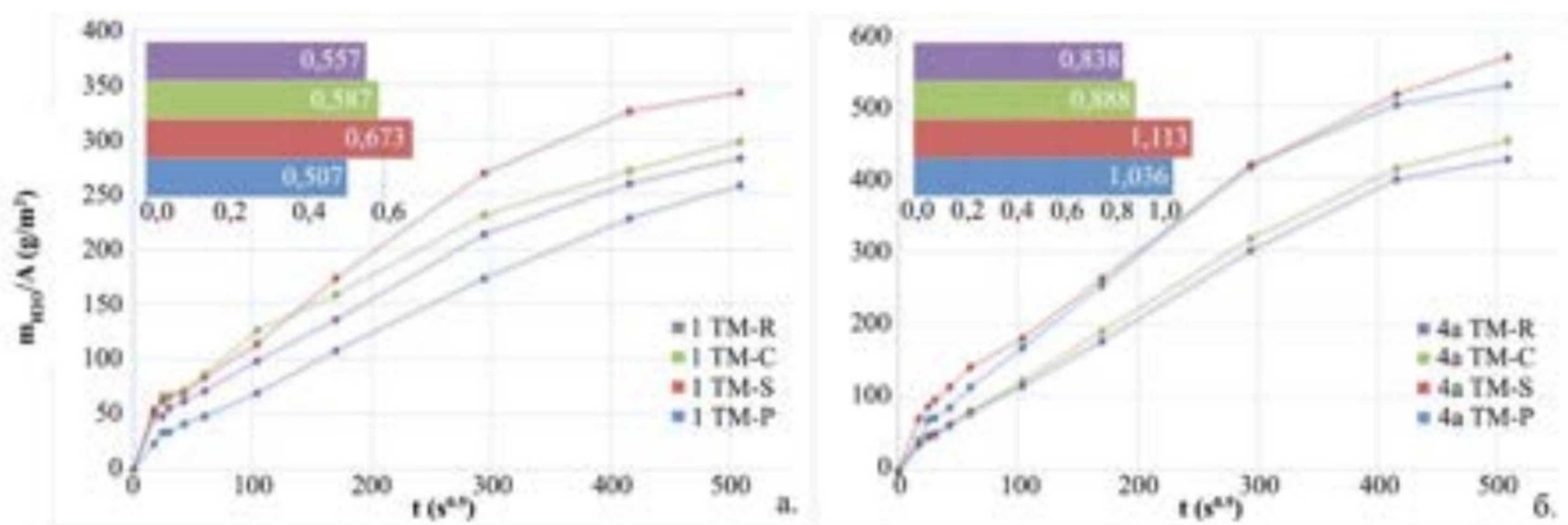
Слика 112. Графички приказ резултата капиларног упијања воде узорка керсантита из каменолома; хистограм коефицијента капиларног упијања воде (C) (горњи леви угао дијаграма) и криве капиларног упијања керсантита узорка а) 1TM и узорка б) 4aTM
