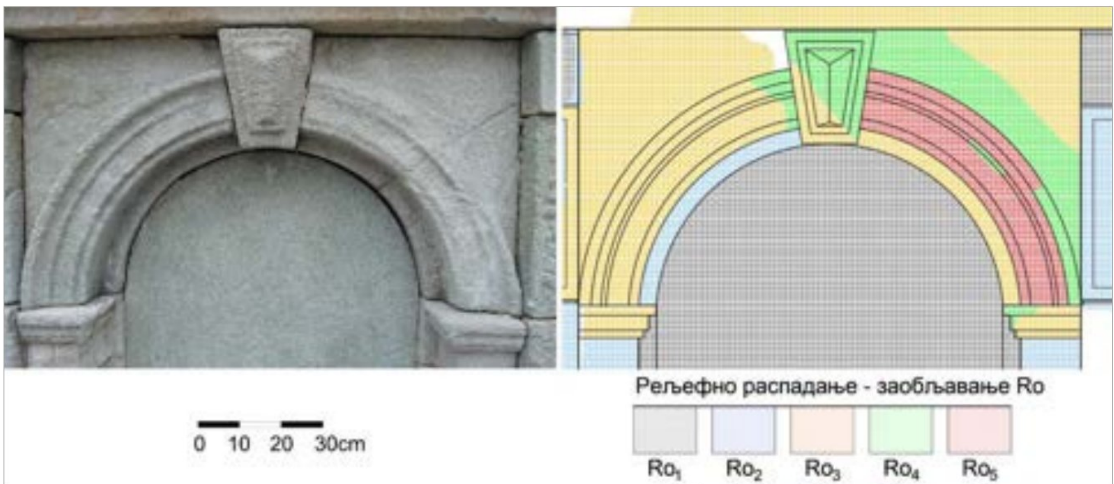
Слика 36. Релјефно распадање: фотографија и графички приказ мапирања
