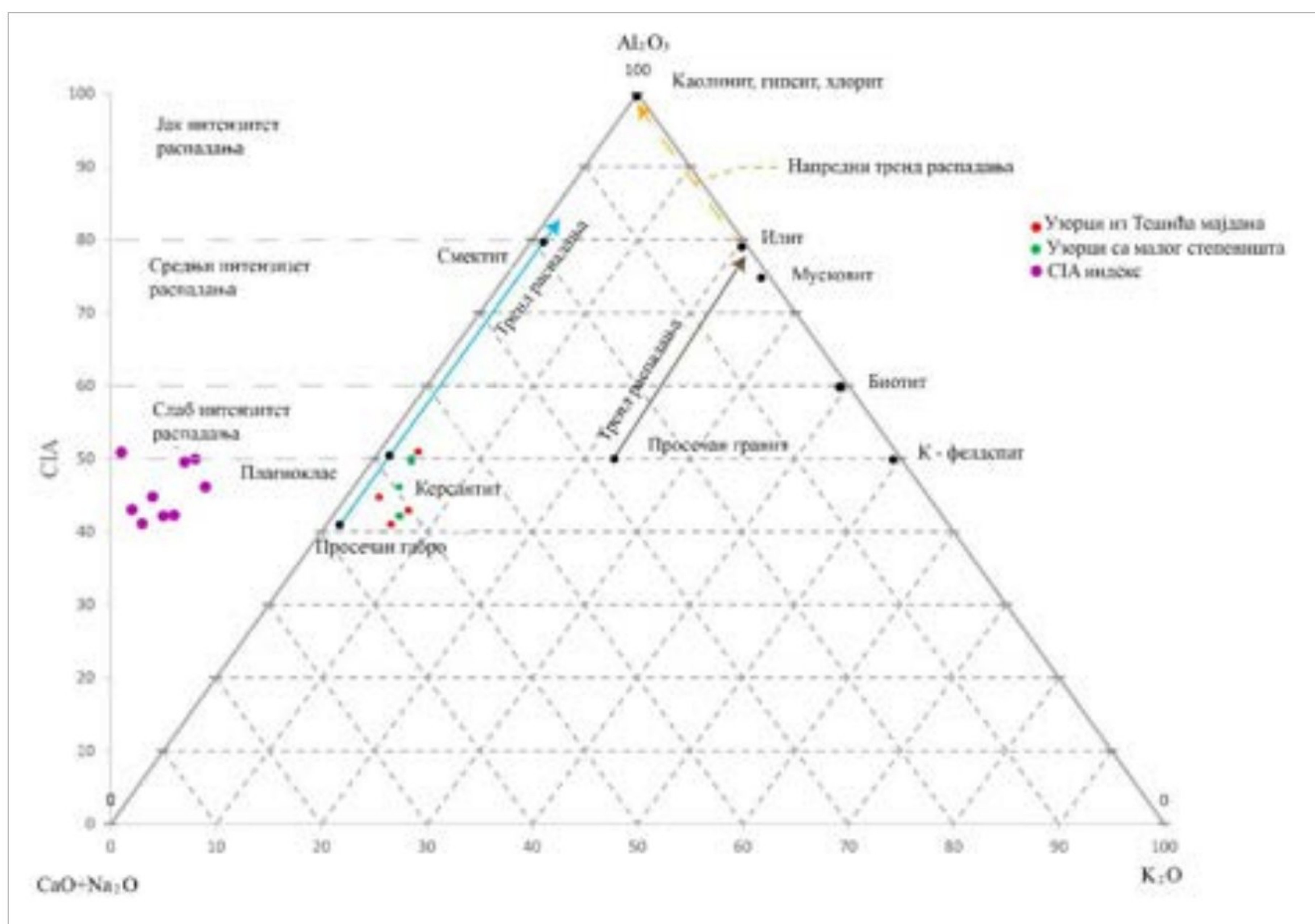
Слика 98. Положај узорака керсантита из каменолома (5TM, 6TM, 7TM и 11TM) и са Малог степеништа (4MS, 6MS, 9MS, 19MS и 20MS) на дијаграму Al_2O_3 , (CaO + Na_2O) , K_2O са упоредним приказом вредности CIA индекса узорака керсантита, наглашеним трендовима распаѓања и диспозицијом минерала (према Nesbitt and Young (1982, 1984, 1989))
