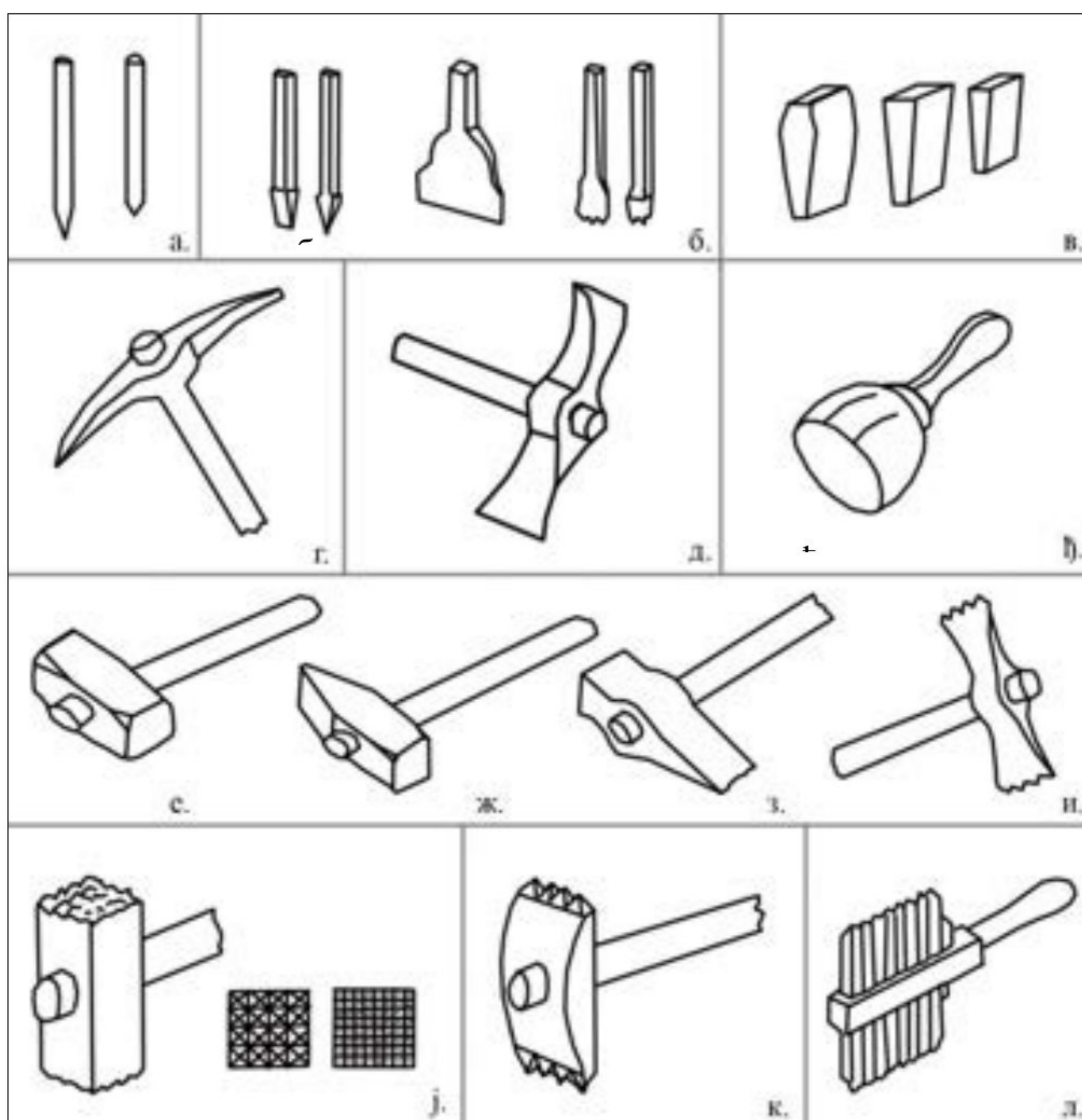
Слика 8. Скице алата за ручну површинску обраду камена а) шпигеви; б) равна и назубљена длета; в) клинови; г) пијук (двошиљак) д) равна секира; е) маљ (дрвени); ж) чекић; з) чекић за босирање; и) назубљена секира; ј) бодљикави чекић за штоковање; к) зубача; л) грелела (модификовано, Pletikosić, 2007)
