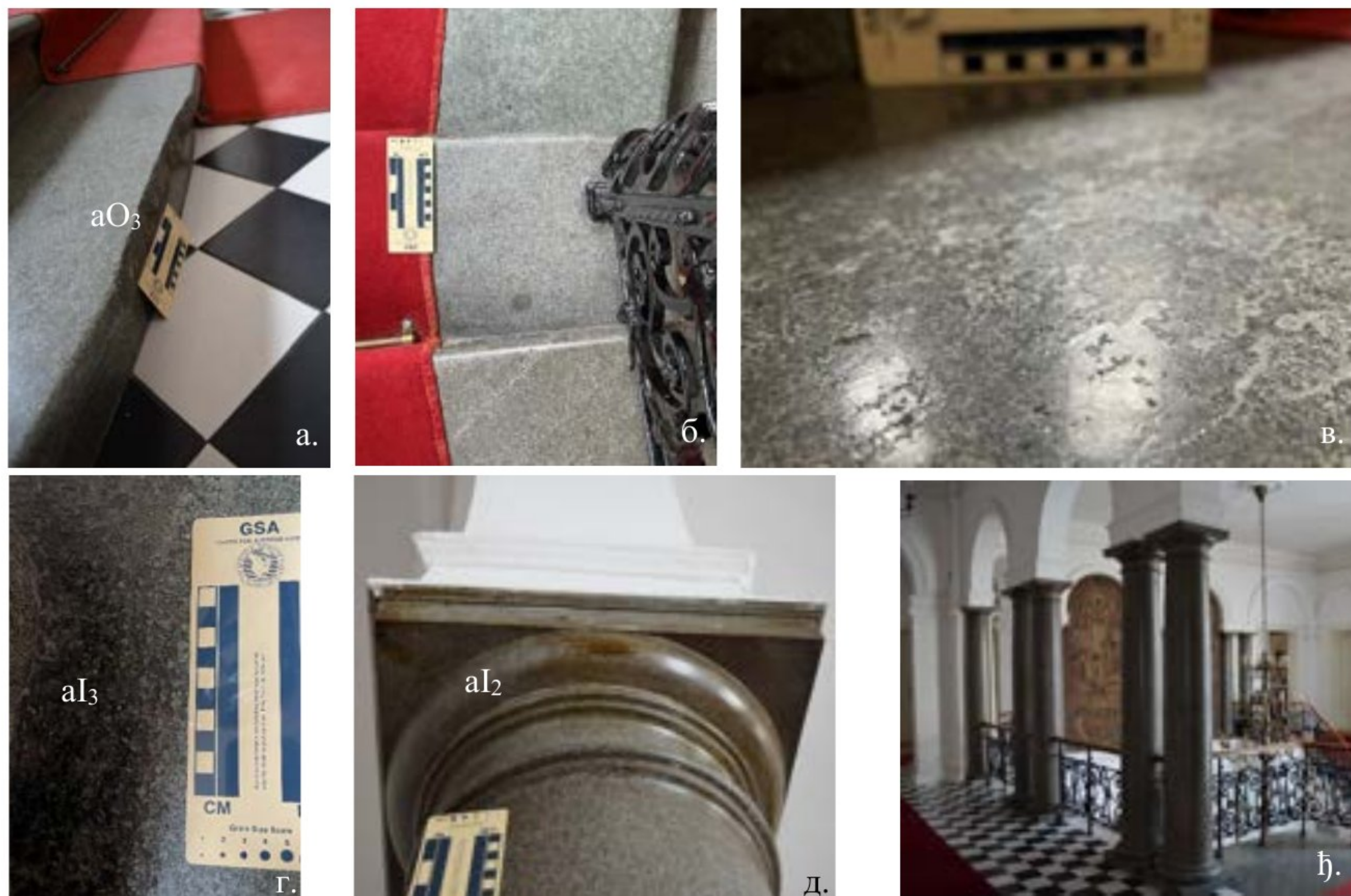
Слика 68. Детаљи ентеријера објекта а) комадасто оштећење првог степеника; б) различити варијетети употребљени за изградњу степеника; в) љускање микрофилма на степеницима; г) запрљање таложјењем средства за заштиту или одржавање; д) запрљање капитета стубова; њ) ентеријер хола на спрату
