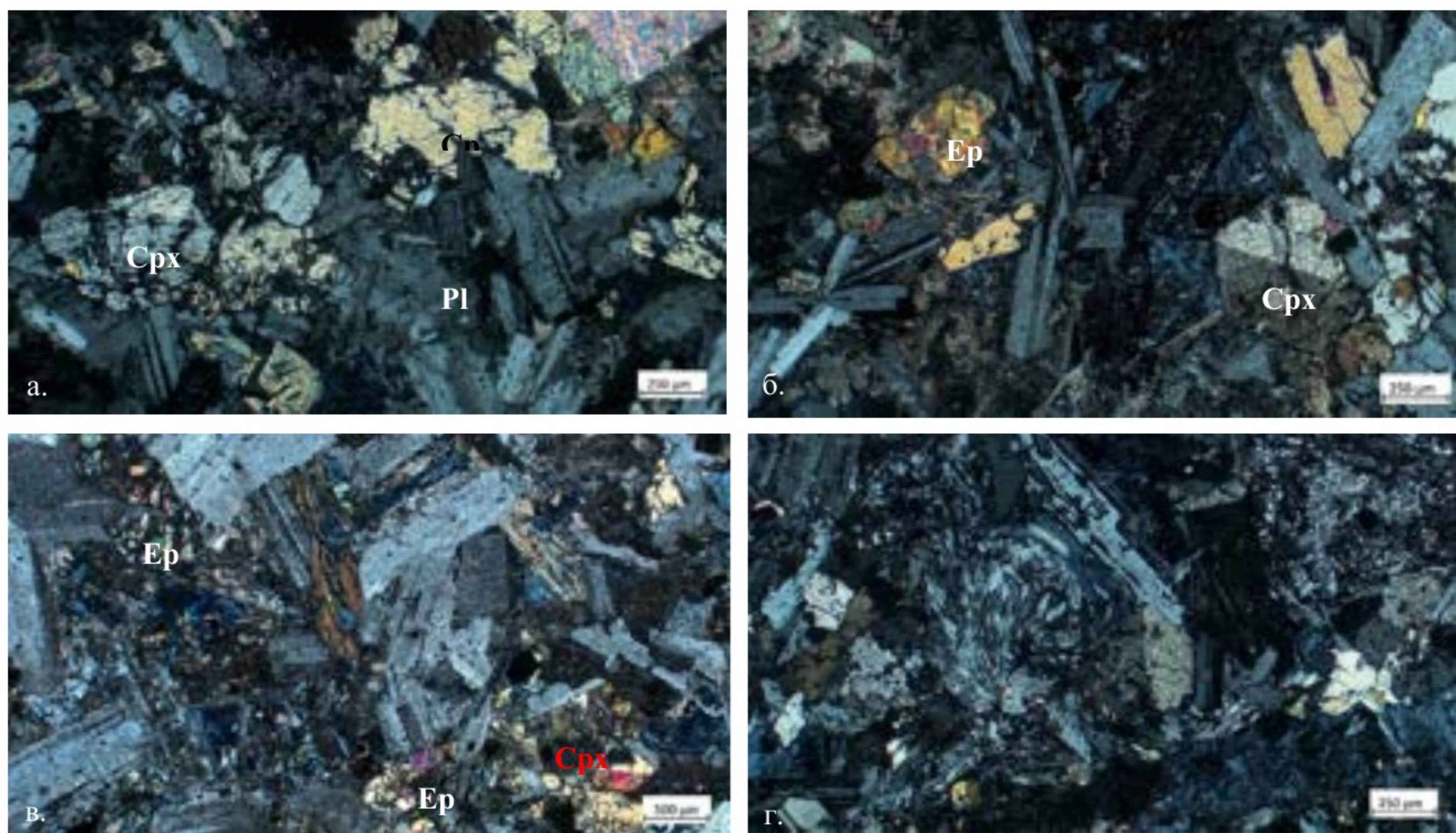
Слика 85. Микрофотографије плагиокласа и пироксена у крупнозрном керсантиту: а) хипидиоморфна алтерисана и испуцала зрна моноклиничних пироксена у узорку 8ТМ, XPL; б) идиоморфна до хипидиоморфна испуцала зрна моноклиничних пироксена, алтерација у епидот и калцит – узорак 8ТМ, XPL; в) реликти пироксена трансформисани у агрегате епидота и калцита – узорак 10ТМ, XPL; г) серпентинисан оливин у крупнозрном керсантиту, узорак 11ТМ, XPL; Легенда ознака: Pl – плагиоклас; Срх – моноклинични пироксен; Ep - епидот
