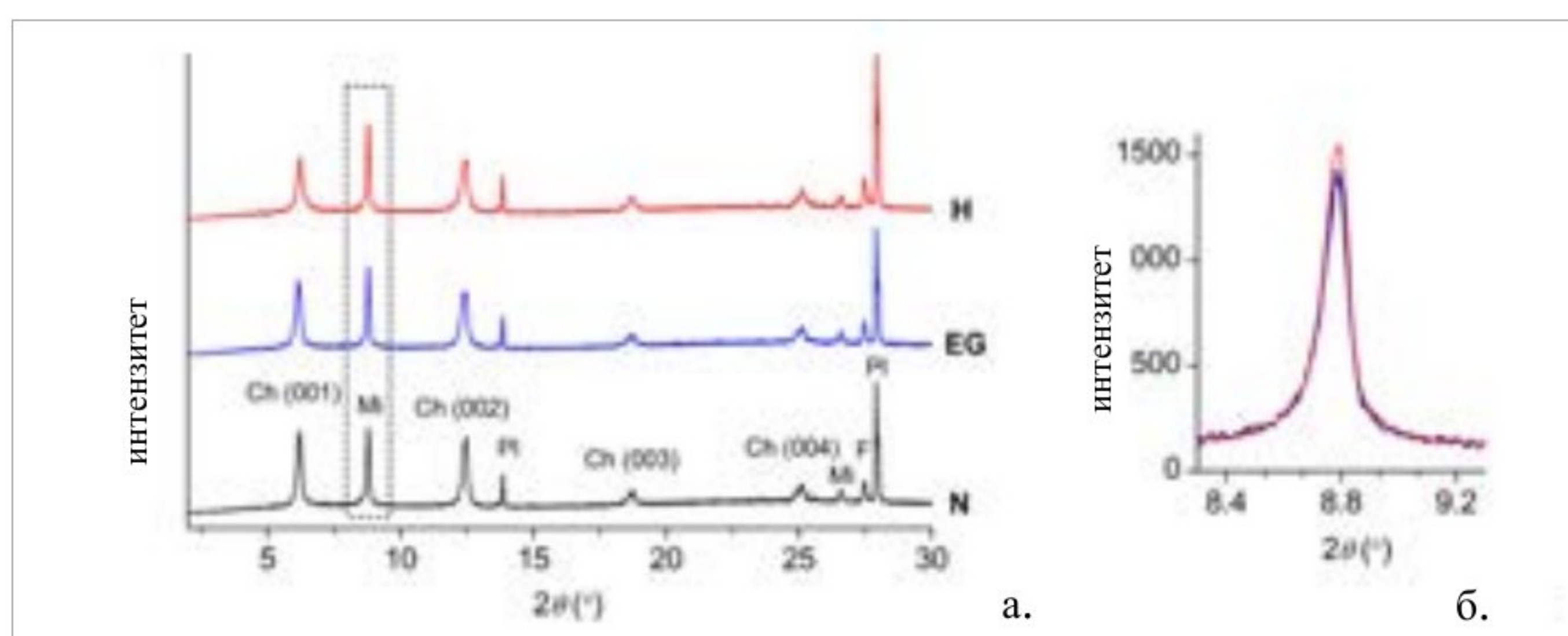
Слика 103. а) Дифрактограми орјентисаних препарата припремљених од узорка 9MS: нетретиран (N), после третмана етилен гликолом (EG) и после загревања (H). Легенда: Ch – хлорит, Mi – лискун, Pl – плагиоклас, F – K-фелдспат, б) преклопљени дифракцијски максимуми (узорак MS 9)
