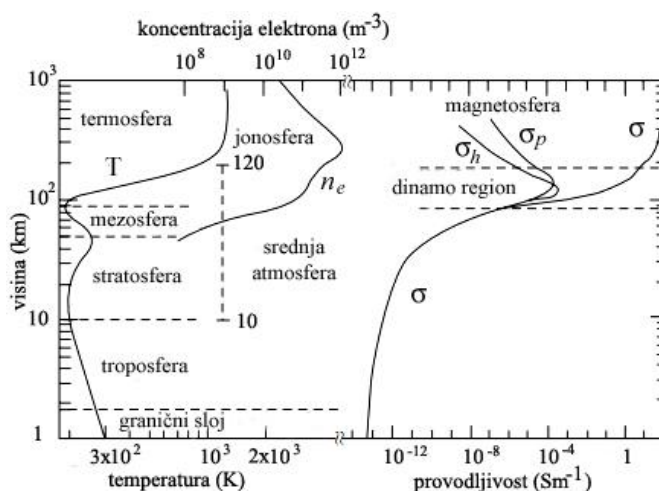
Slika 1.1.1. Varijacije sa visinom najvažnijih parametara atmosfere i jonosfere (Hargreaves, 1992)
