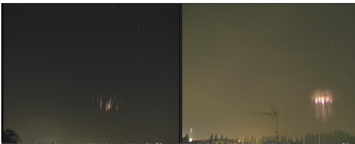
c) klaster, kolumn sprajtovi
