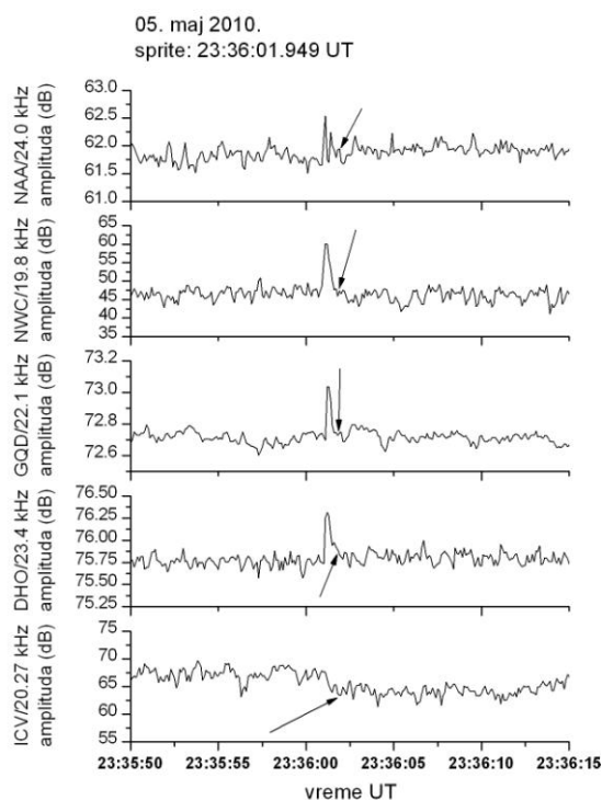
Slika 6.1.3. Primer kada pojava atmosferskog pražnjenja prethodi pojavi sprajta dok VLF poremećaj koji pripada istoj olujnoj aktivnosti započinje ranije (vreme sprajta obeleženo je strelicom)
