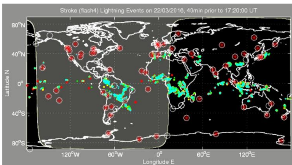
Slika 4.1.1.1. Lokacije atmosferskih pražnjenja registrovane WWLLN mrežom ( http://wwlln.net/new/ )
