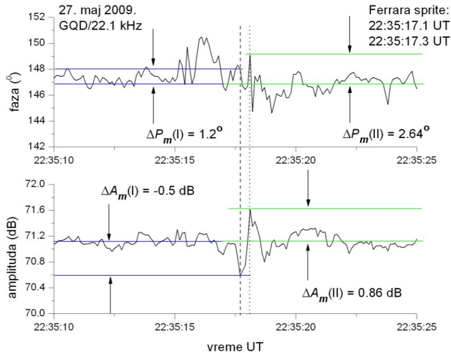
Slika 6.2.1.2. Određivanje izmerenih vrednosti \Delta A_m i \Delta P_m u slučaju GQD/22.1 kHz signala
