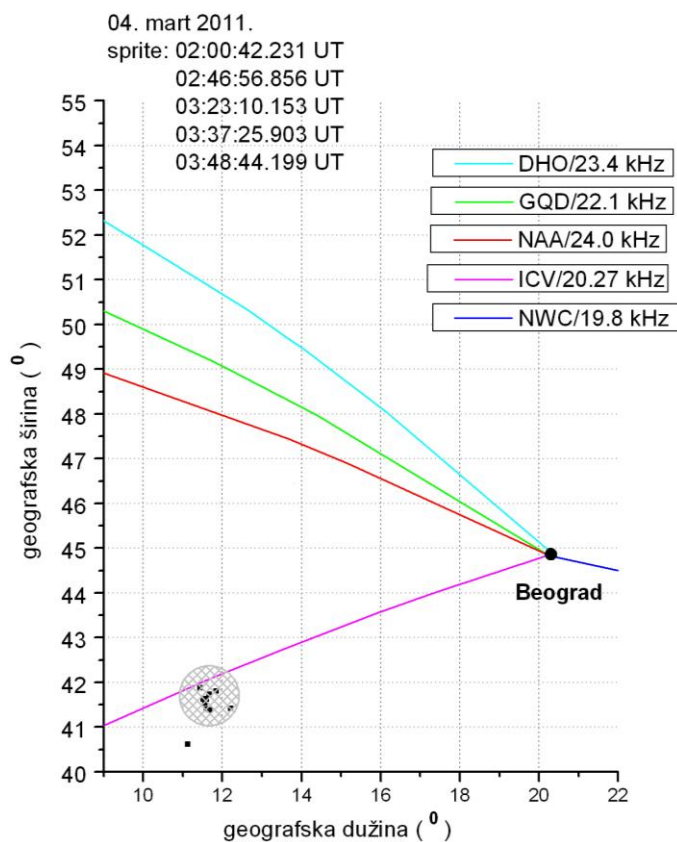
Slika 6.2.2.4. Pretpostavljeni položaj jonosferske neregularnosti u slučaju LORE poremećaja registrovanih na ICV/20.27 kHz trasi 04. marta 2011. godine prikazan je sivom elipsom (atmosferska pražnjenja prikazana su crnim kvadratićima)
