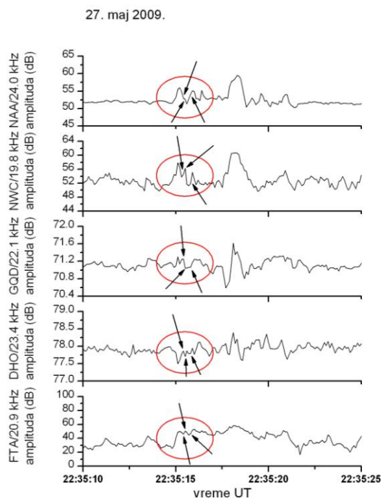
Slika 6.1.7. Primer kada pojava atmosferskog pražnjenja prethodi VLF poremećaju zaokruženom crvenom bojom i sprajt nije zabeležen kamerama I.M.T.N. mreže (vremena atmosferskih pražnjenja registrovanih mrežom EUCLID obeležena su strelicama)
