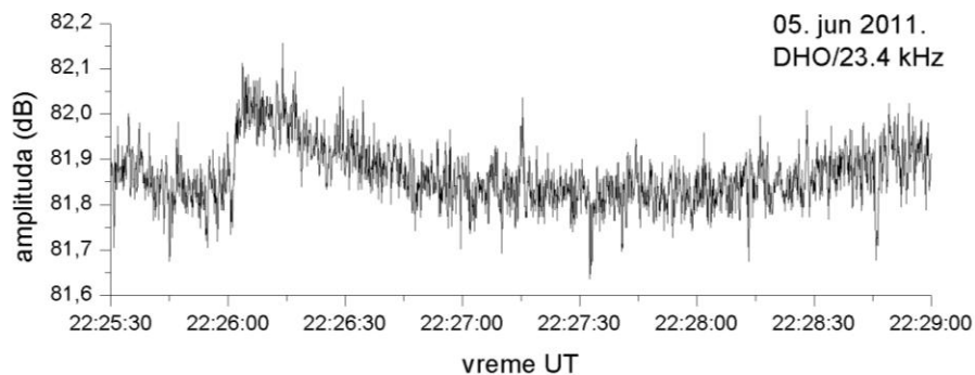
Slika 6.1.9. Tipičan LEP poremećaj
