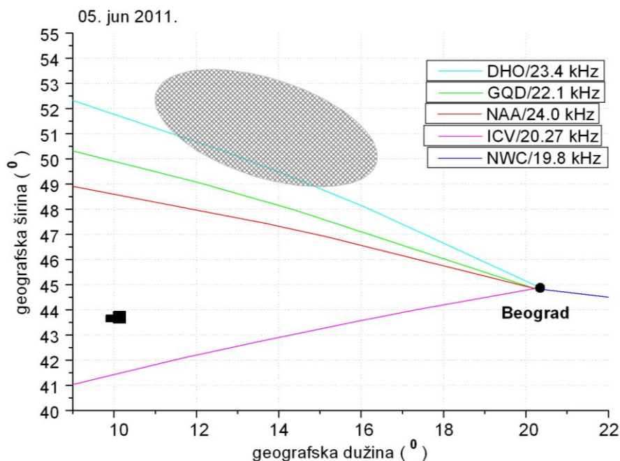
Slika 6.1.10. Pretpostavljeni položaj LIE u slučaju LEP poremećaja registrovanog 05. juna 2011. godine obeležen je sivom elipsom (atmosferska pražnjenja predstavljena su crnim kvadratićima)
