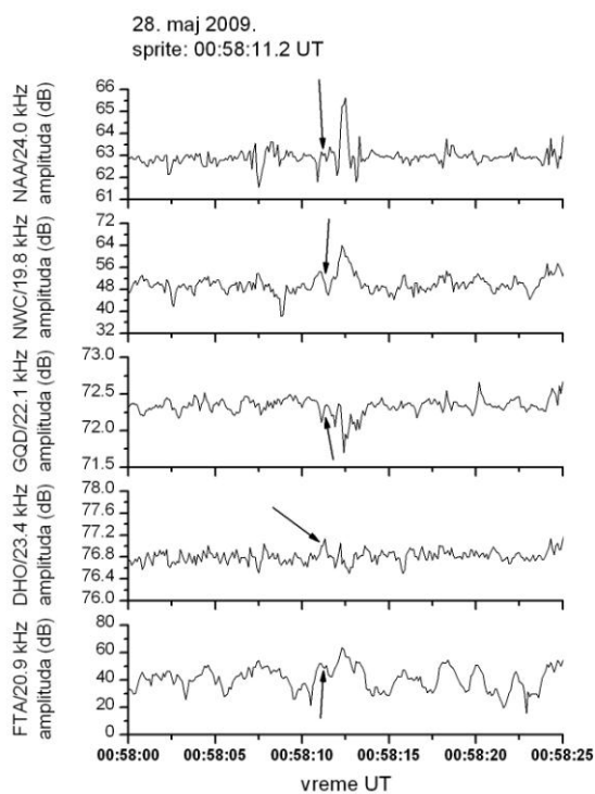
Slika 6.1.4. Primer kada pojava sprajta prethodi VLF poremećaju dok atmosfersko pražnjenje prema informacijama pomenutih mreža nije zabeleženo (vreme sprajta obeleženo je strelicom)
