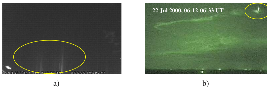
Slika 2.5.1. Snimci pražnjenja iznad vrha oblaka naviš:
