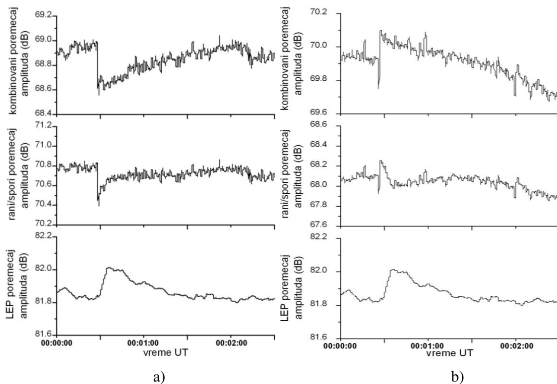
Slika 6.1.11. Sintetički kombinovani VLF poremećaji dobijeni superponiranjem izgladenog ranog/sporog i LEP poremećaja
