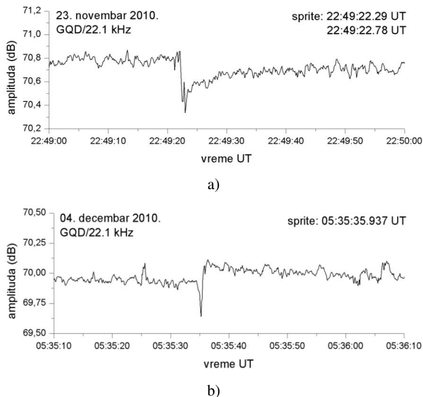
Slika 6.1.8. Tipični VLF poremećaji kombinovani od ranih/sporih i LEP poremećaja
