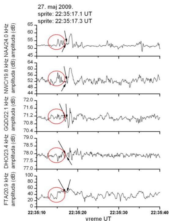
Slika 6.1.2. Primer kada pojava atmosferskog pražnjenja prethodi pojavi sprajta koji prethodi VLF poremećaju (vremena sprajtova obeležena su strelicama)
