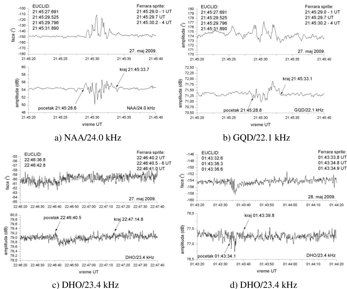
Slika 6.2.1. Razvoj VLF poremećaja u odnosu na vremena zabeleženih sprajtova i atmosferskih pražnjenja tokom noći 27 - 28. maja 2009. godine
