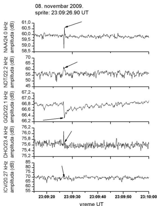
Slika 6.1.6. Primer kada pojava VLF poremećaja prethodi pojavi sprajta dok atmosfersko pražnjenje prema informacijama pomenutih mreža nije zabeleženo (vreme sprajta obeleženo je strelicom)
