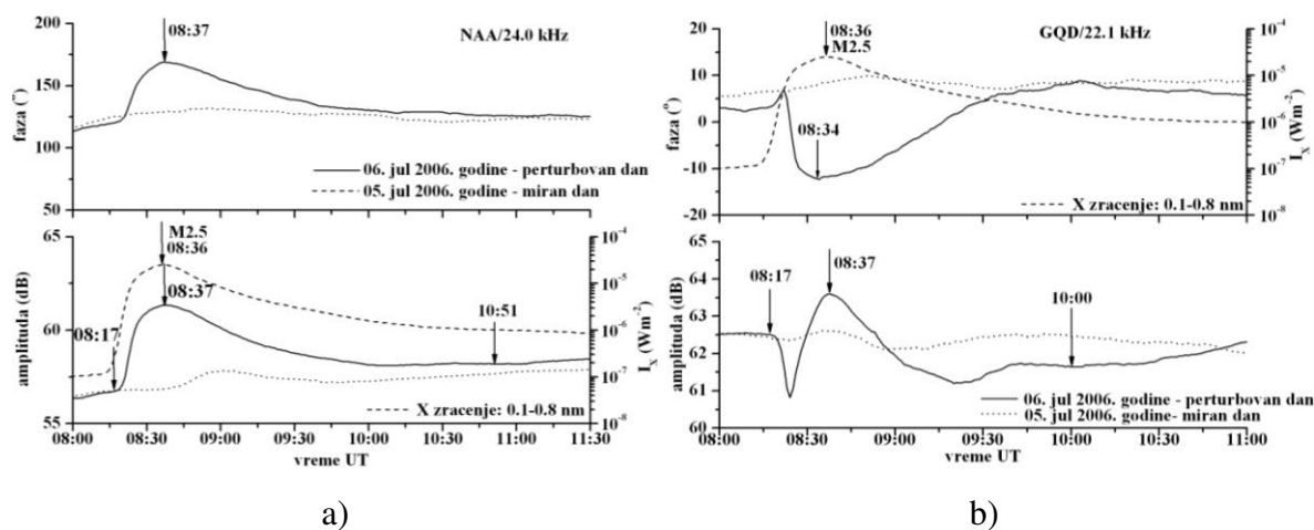
Slika 6.2.1.5. Poremećaj dnevnog VLF signala tokom maksimuma X-zračenja solarnog flera klase M2.5 registrovanog 06. jula 2006. godine u 08:36 UT na trasi:
