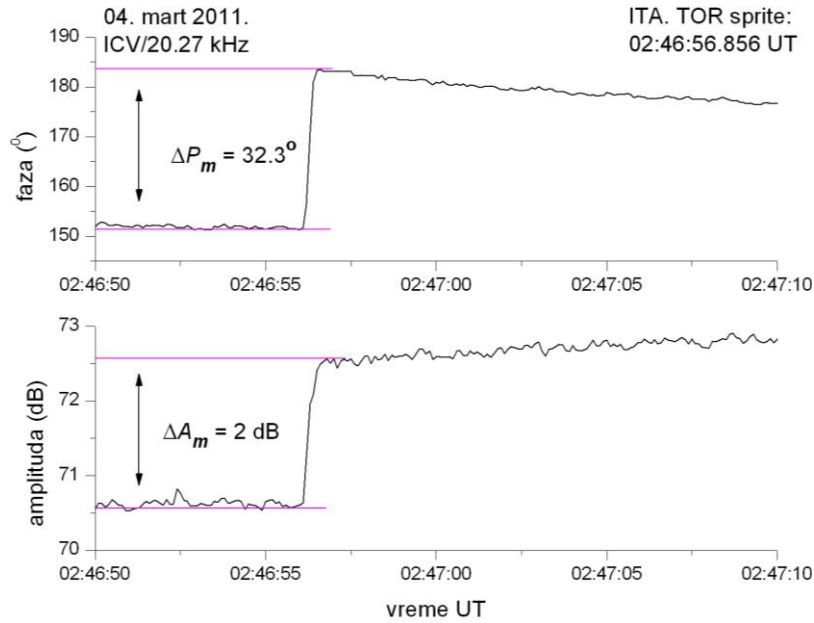
Slika 6.2.2.3. Određivanje izmerenih vrednosti \Delta A_m i \Delta P_m u slučaju ICV/20.27 kHz signala
