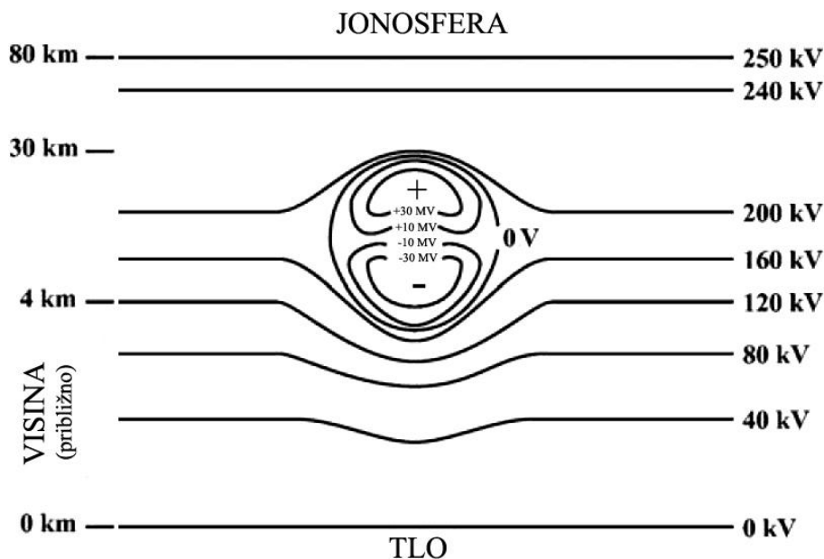
Slika 1.3.3.1. Dijagram raspodele ekvipotencijalnih površi između Zemlje i jonosfere u blizini idealizovanog olujnog oblaka pre pojave atmosferskog pražnjenja (Füllekrug et al. eds, 2006)
