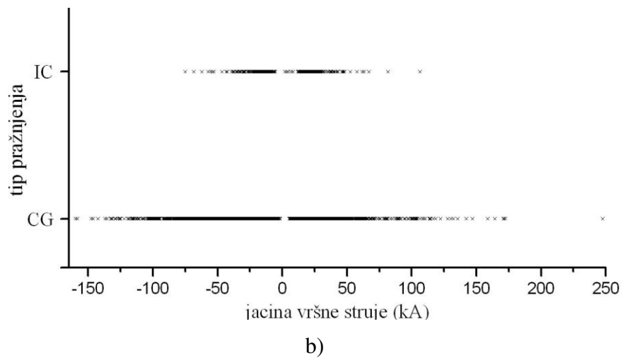
Slika 6.2.1.3. Olujna aktivnost zabeležena EUCLID mrežom iznad područja ograničenog koordinatama 12 I - 22 I i 40 S - 48 S tokom noći 27 - 28. maja 2009. godine: a) zabeležena atmosferska pražnjenja i pripadajuće jačine vršnih struja i b) zabeleženi tipovi atmosferskih pražnjenja i pripadajuće jačine vršnih struja
