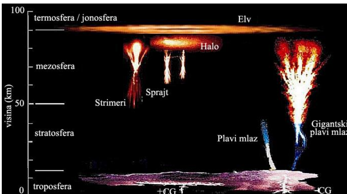
Slika 2.1. Shematski prikaz osnovnih tipova TLE pojava
