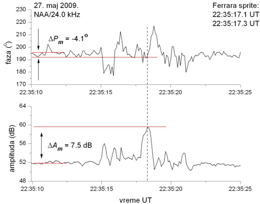
Slika 6.2.1.1. Određivanje izmerenih vrednosti \Delta A_m i \Delta P_m u slučaju NAA/24.0 kHz signala
