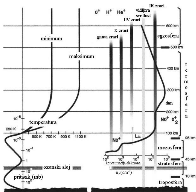
Slika 1.1.2. Atmosferske i jonosferske oblasti (Goodman, 2005)
