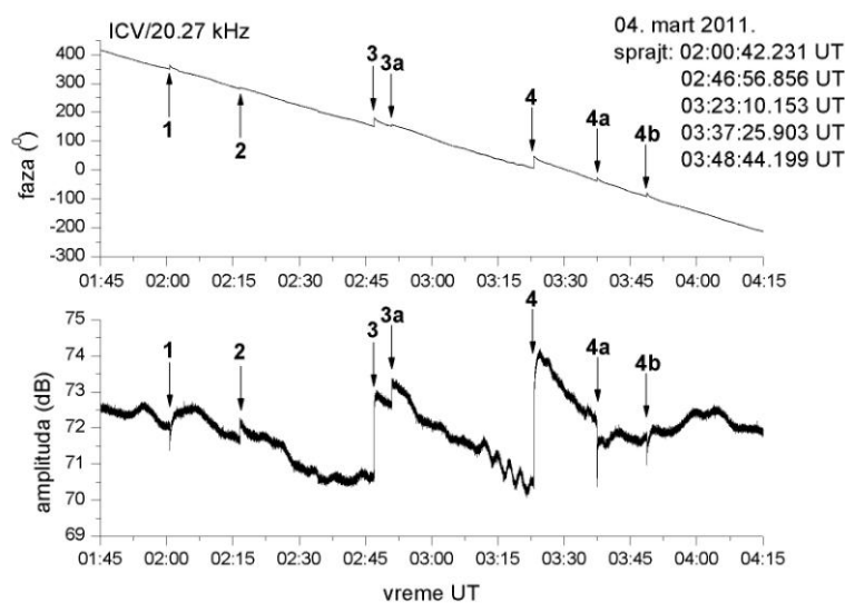
Slika 6.2.2.1. Poremećaji prostiranja ICV/20.27 kHz signala u slučaju pojave elva sa sprajtovima registrovani 04. marta 2011. godine
